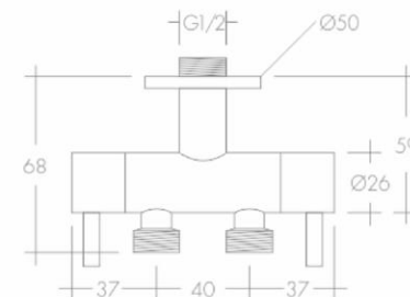
TORNEIRA ESQUADRIA DUPLA CROMADA PRINT (Ø1/2 x 1/2 x 1/2)
